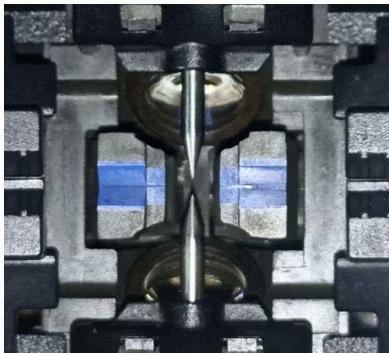
Img 2 Cambio de electrodos
