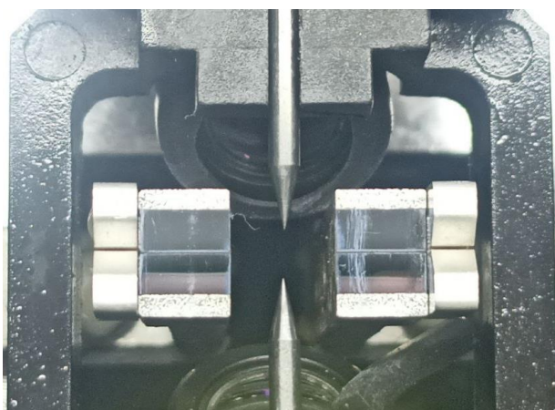
Img 3 Cambio de electrodos
